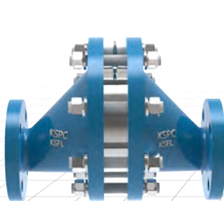
KSFL type
